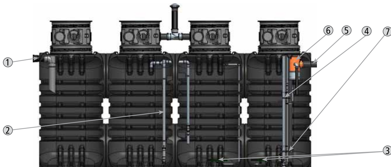
Vue de coupe d'une micro-station ACTIBLOC® 12EH (10000 SP).
