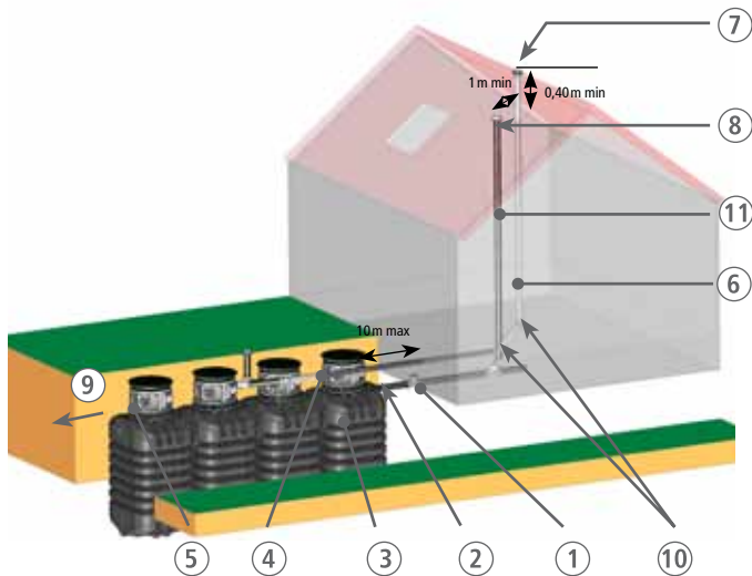
Schéma de raccordement de la ventilation haute pour une micro-station ACTIBLOC® 12EH (10000 SP).
