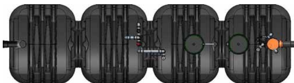
Vue de coupe d'une micro-station ACTIBLOC® 12EH (10000 SP).
