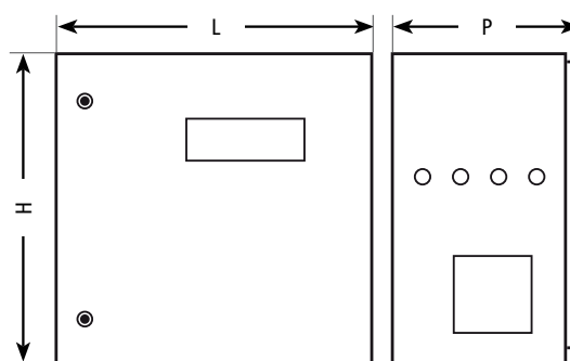
Dimensions de l'armoire intérieure métallique (Art. : 32734).
